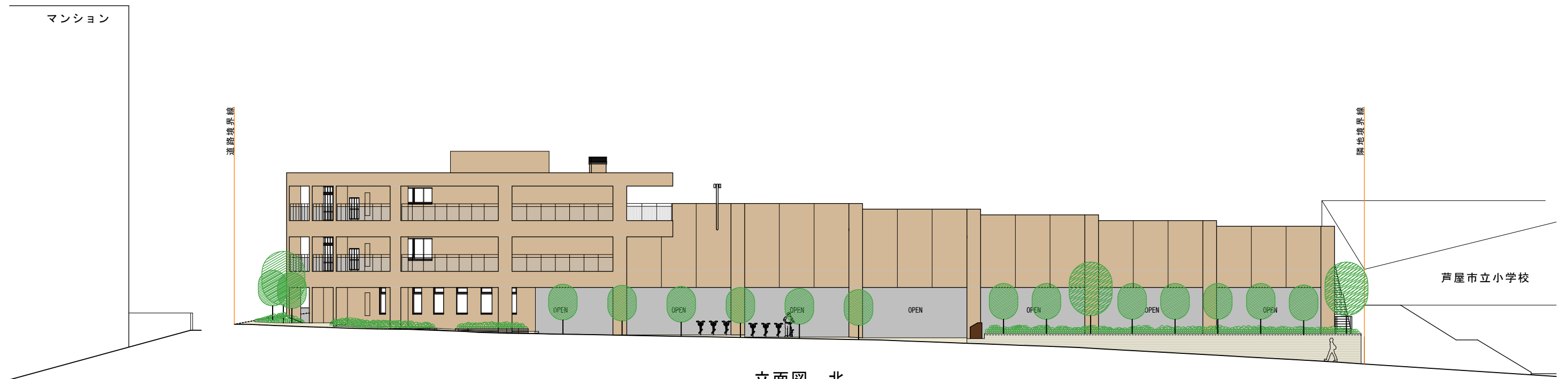
立面図 北
