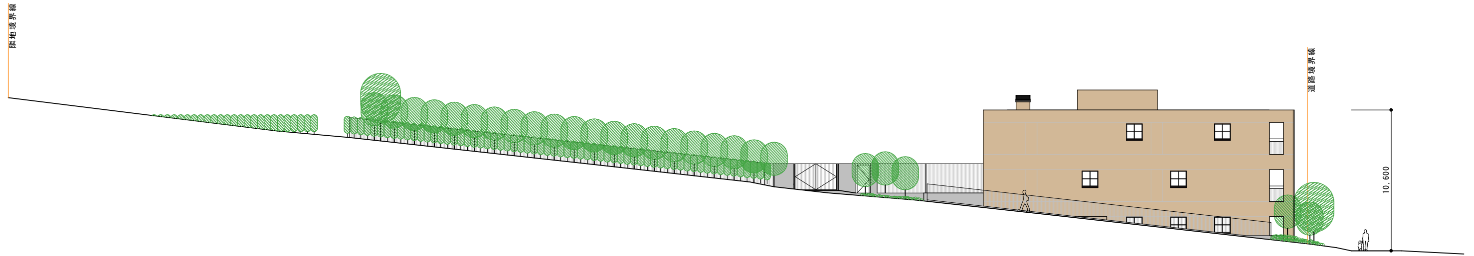
立面図 南
