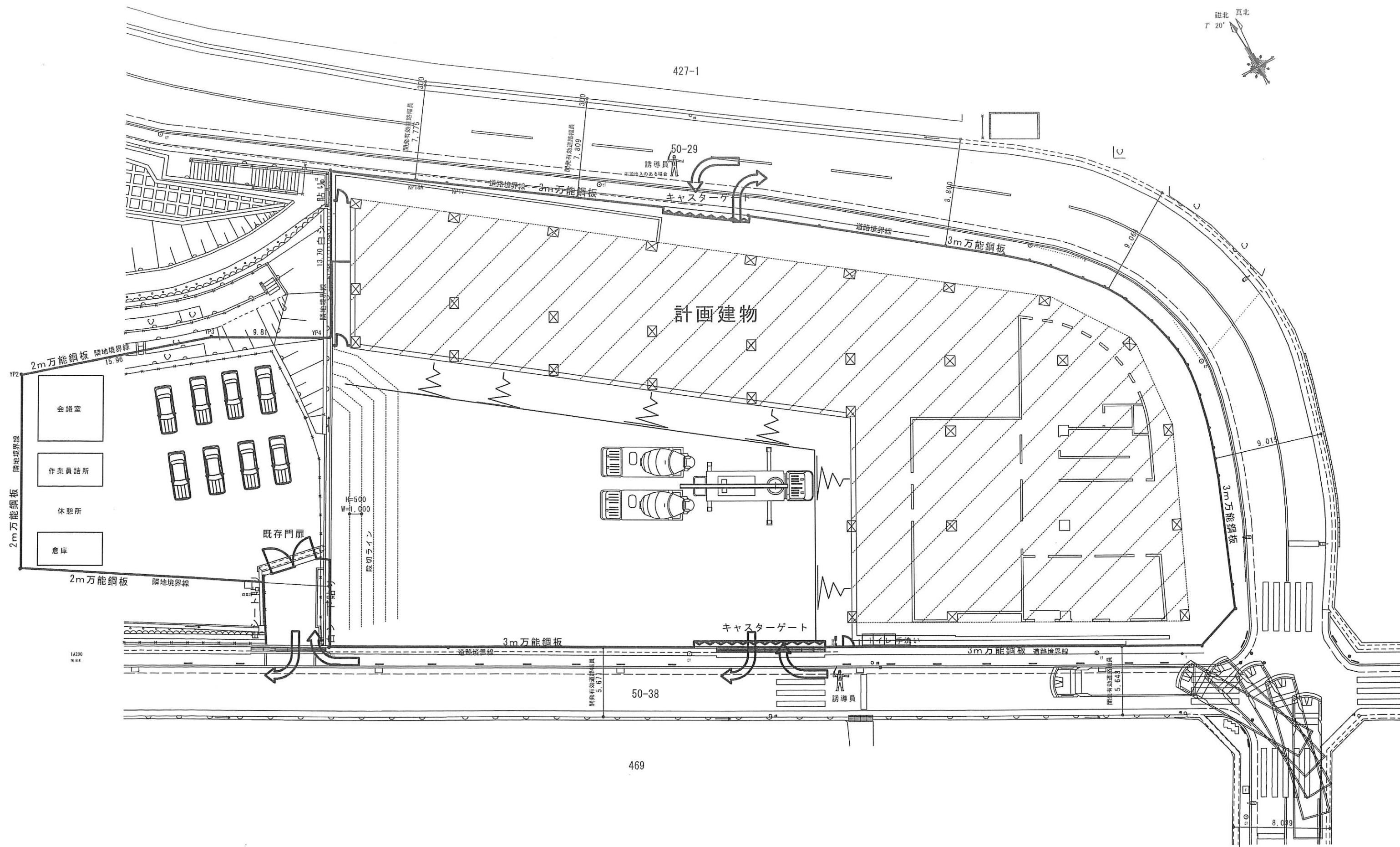
総合仮設図
