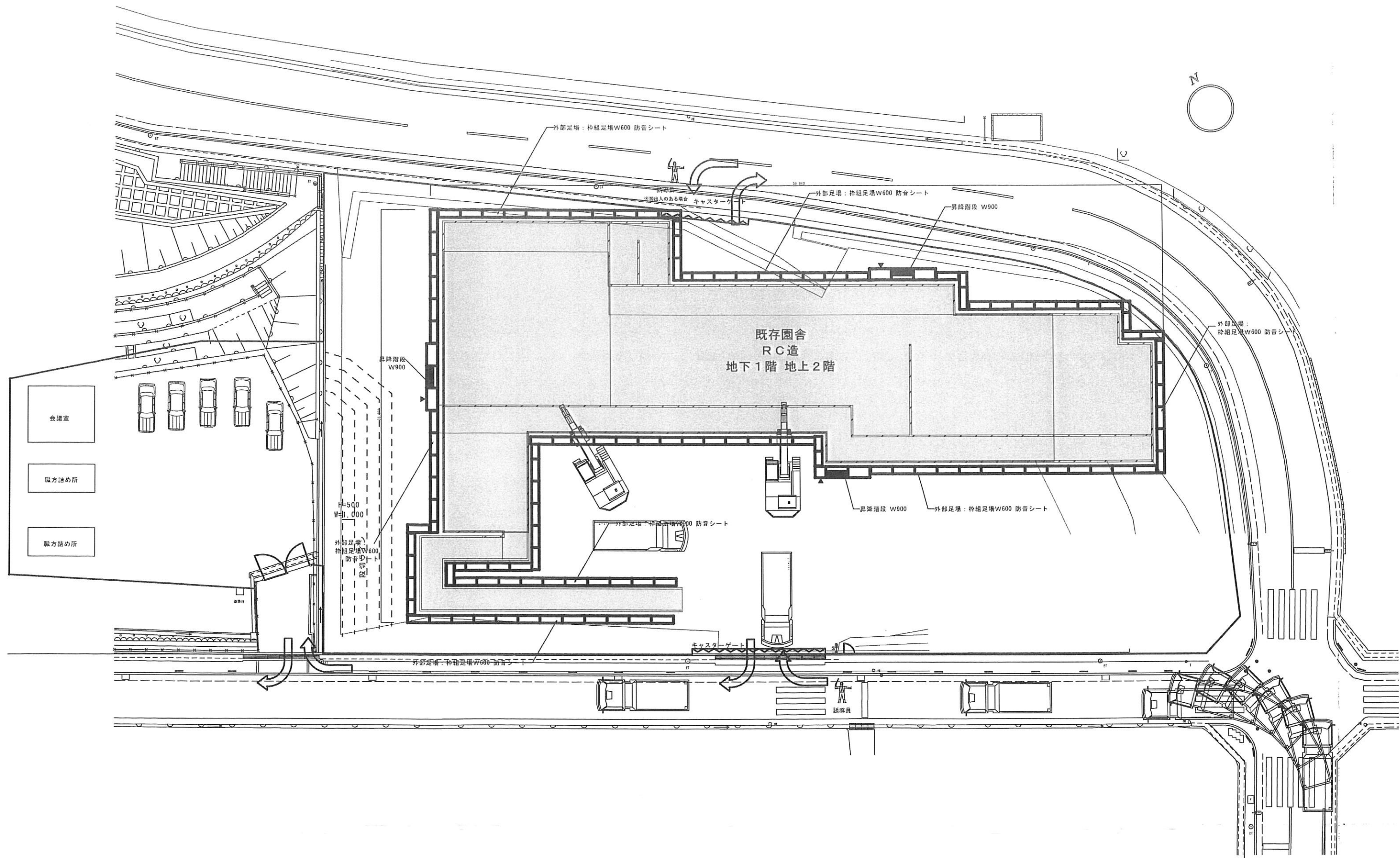
解体仮設総合図
